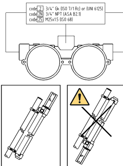
Installazione a palina Pole mounting
