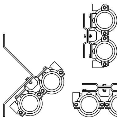
Installazione parete Wall mounting
