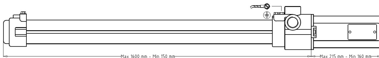
Installazione a sospensione Suspended mounting
