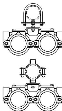
Installazione a palina Pole mounting
