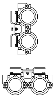
Installazione soffitto e parete Ceiling and wall mounting
